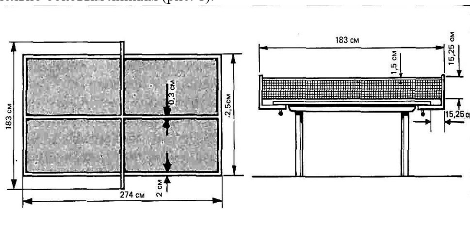
Рис 1. Размеры теннисного стола Игровая площадка, на которой, как правило, размещается стол, имеет размеры для российских соревнований 5 м х 7 м и огорожена бортиками темного цвета высотой 75 см.
